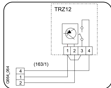
Fig. 8 - Conexión del cronotermostato. (Previamente eliminar puente entre 1 y 4, fig. 7, pos. 163/1)
